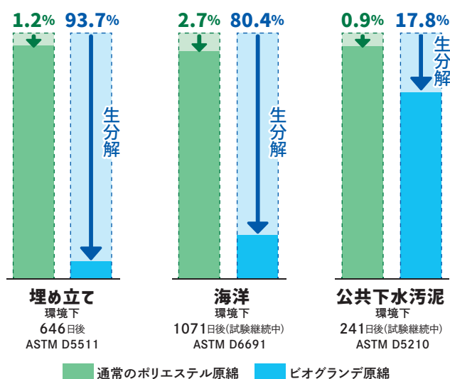
様々な環境下での生分解性試験 (原綿)
